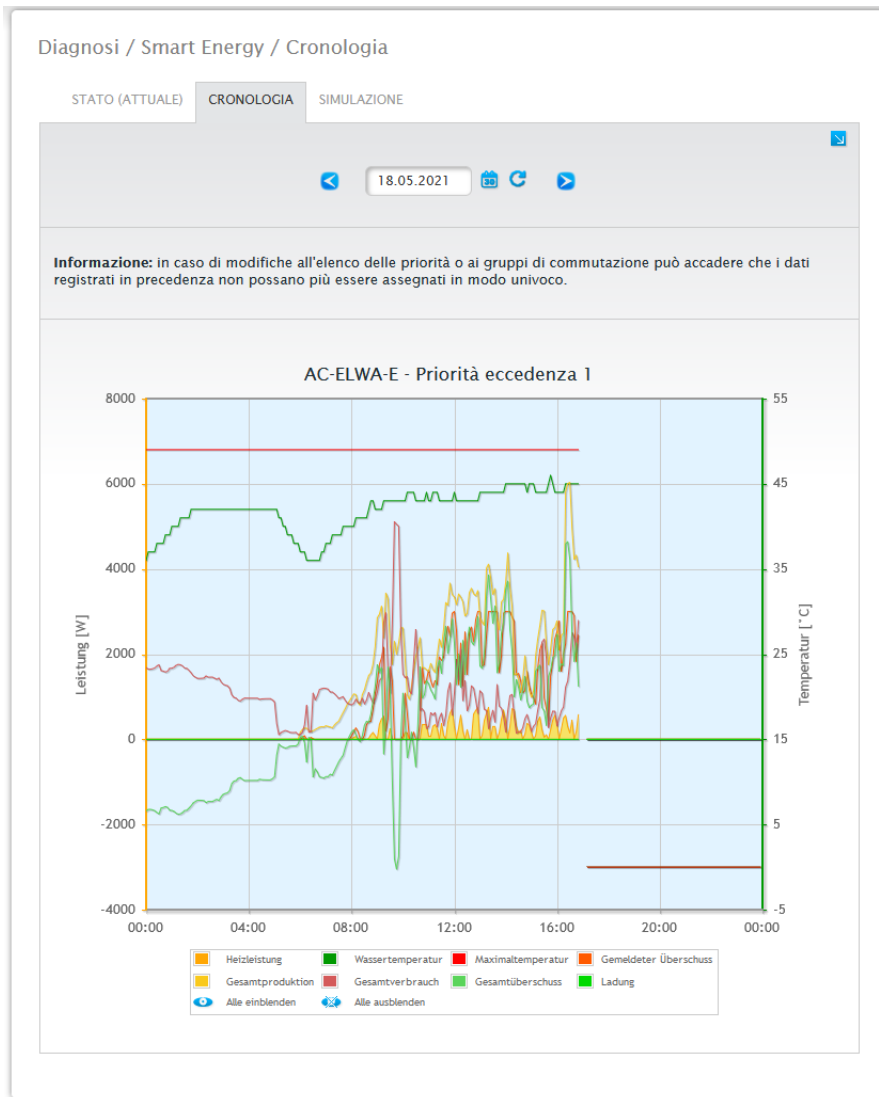
Fig.: Cronologia Smart Energy - Esempio Priorità 1
