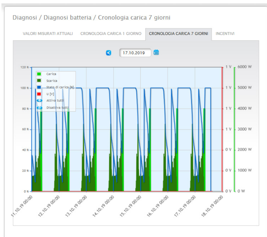
Fig.: Diagnosi batteria - Cronologia carica 7 giorni
