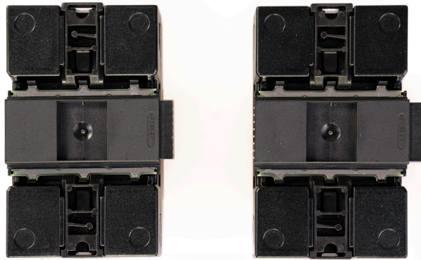
Fig.: Solar-Log Base e Solar-Log MOD I/O con connettore bus
