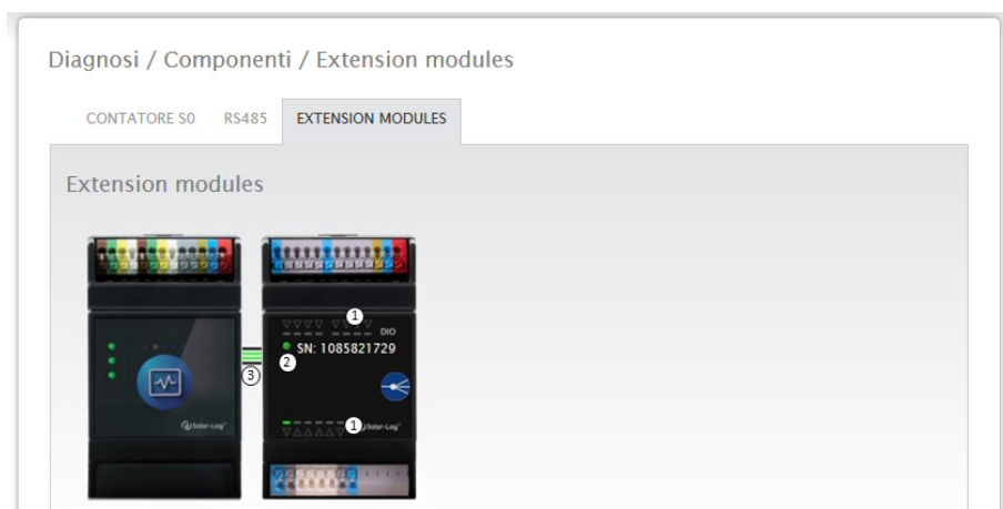
Fig.: Bus di comunicazione/LED Solar-Log MOD I/O - Solar-Log Base
